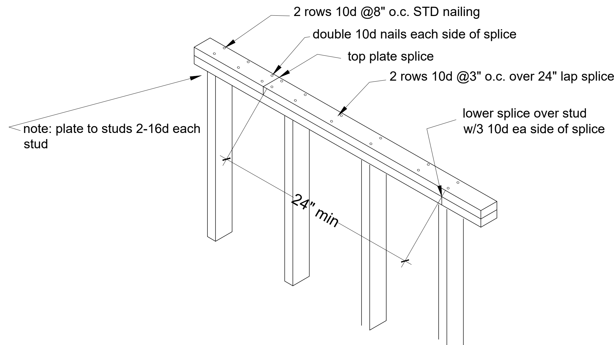
Top Plate Splice Detail Scale: N.T.S.
