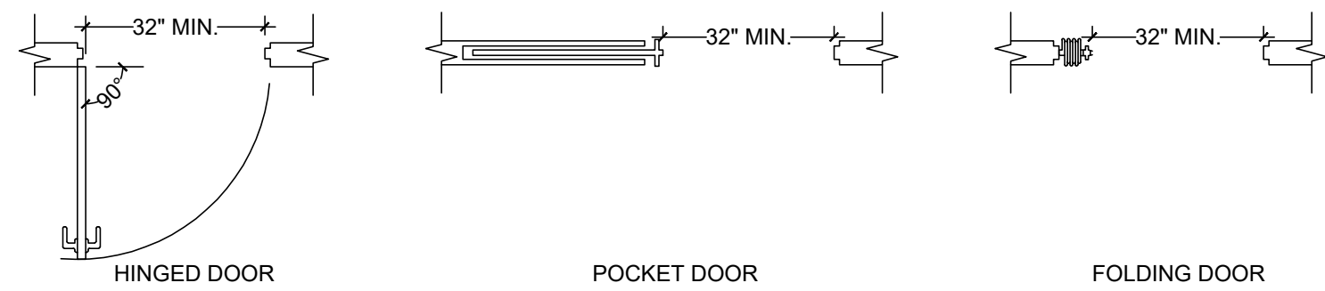
Door Clear Widths Scale: 3/8" = 1'-0"
