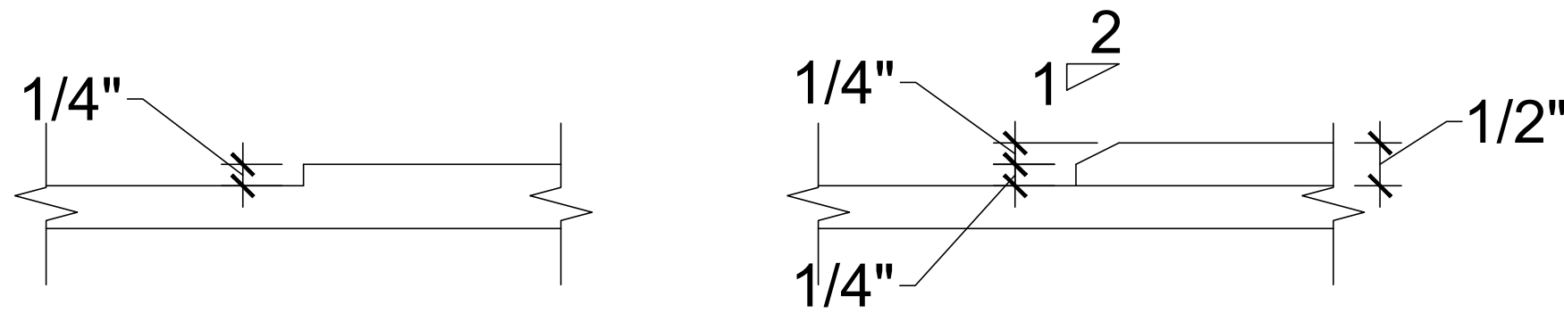
Vertical Change Scale: 6" = 1'-0"
