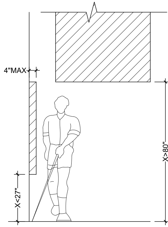
Protruding Object Scale: 3/8" = 1'-0"
