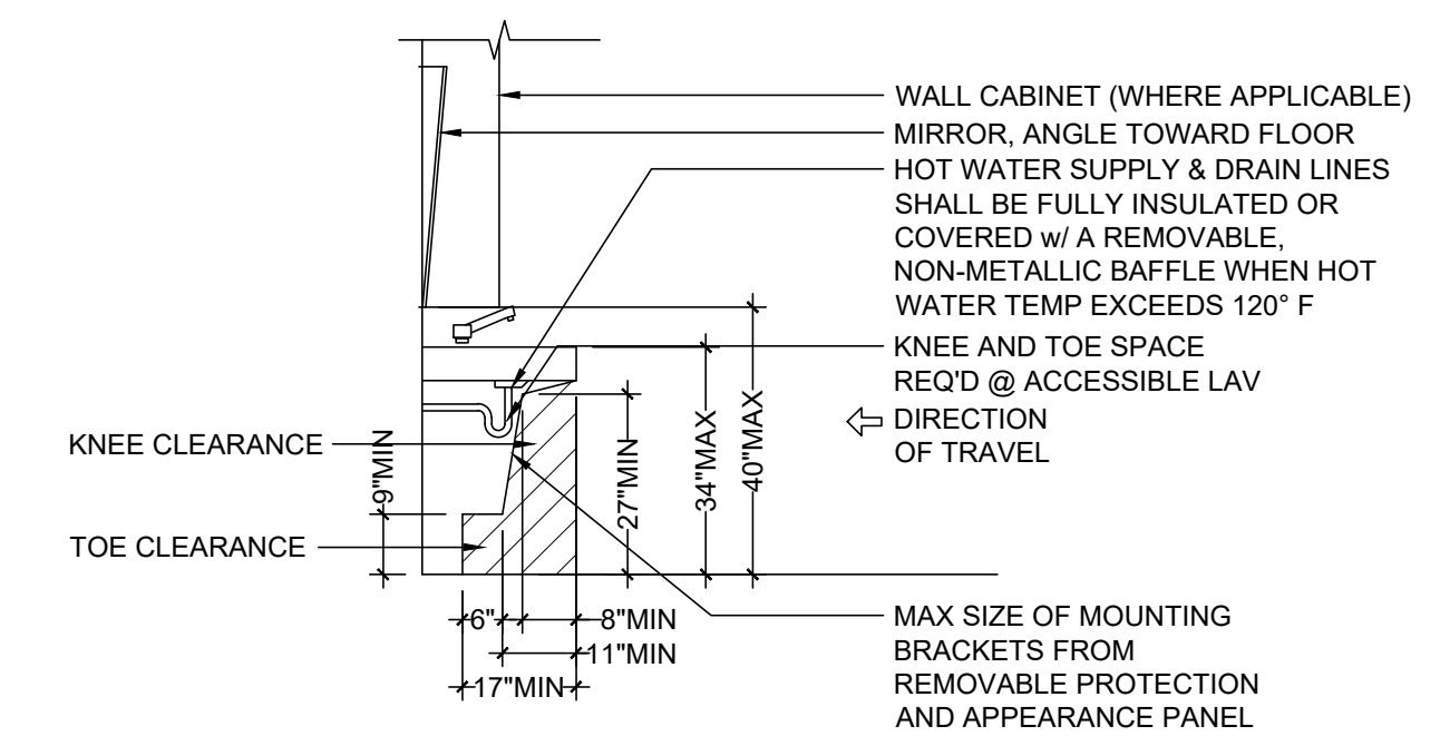
Accessible Sink Scale: 3/8" = 1'-0"
