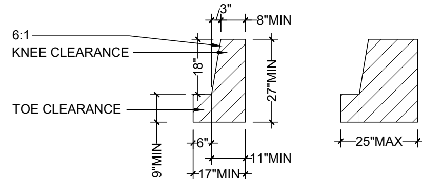
Knee/Toe Clearance Scale: 3/8" = 1'-0"
